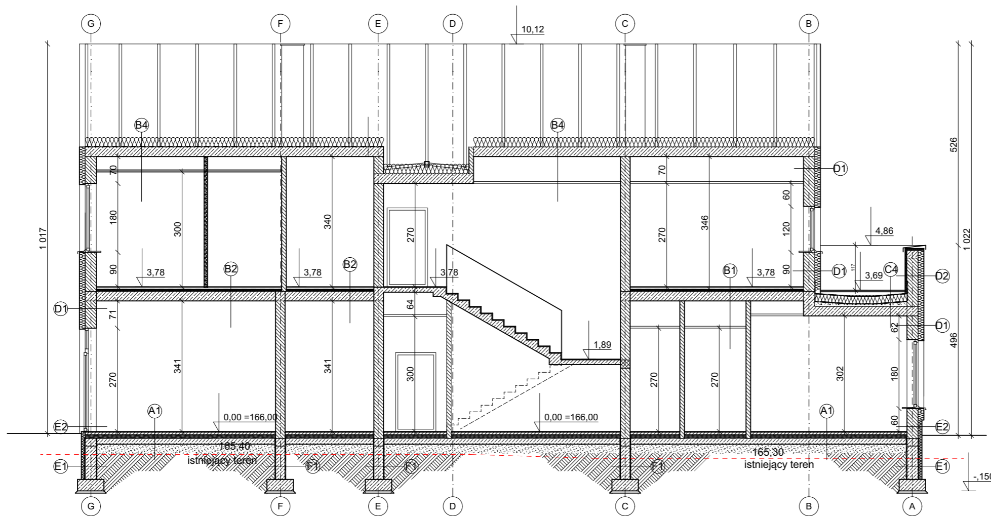
RZEKRÓJ C-C
